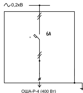
Схема электрическая принципиальная
