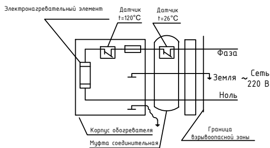
Схема электрических обогревателей ОША-Р-4
