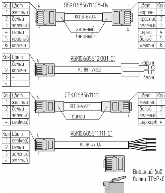
Рисунок Б.4 – Цветовая маркировка проводов кабелей
