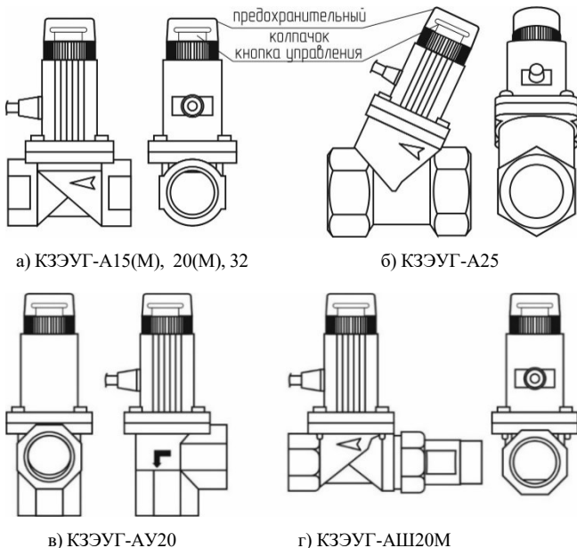
Рисунок 2 – Внешний вид клапанов КЗЭУГ-А
