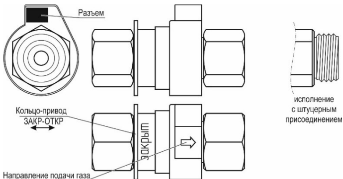
Рисунок 3 – Внешний вид клапана КЗЭУГ-Б
