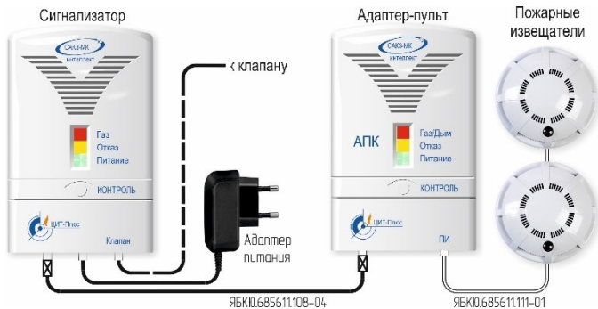
Рисунок Б.2 – Схема соединений с пожарными извещателями
